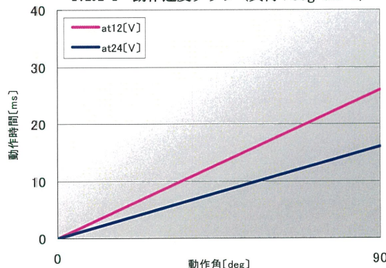
47RT-4 動作速度グラフ (負荷: 80\text{g} \cdot \text{cm}^2 )
